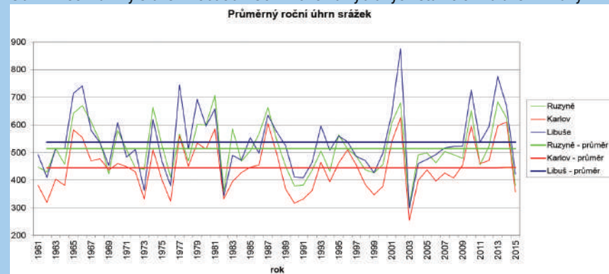
Obr. 4: Roční úhrny srážek v období 1961–2015 na vybraných stanicích na území Prahy
