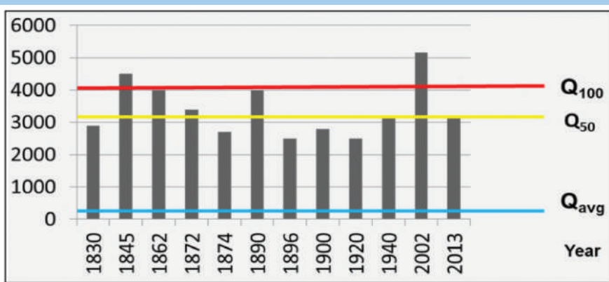
Obr. 7: Povodně na Vltavě v období 1830–2013
