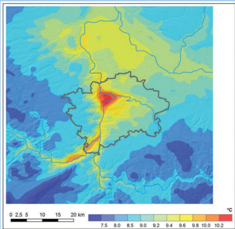
Obr. 3: Průměrná roční teplota v Praze a okolí v období 1961–2013
