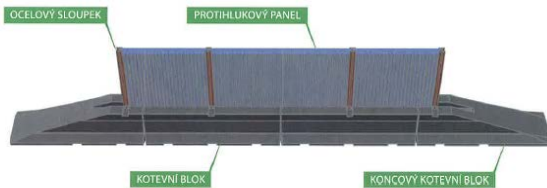
Postup montáže protihlukové mobilní stěny
